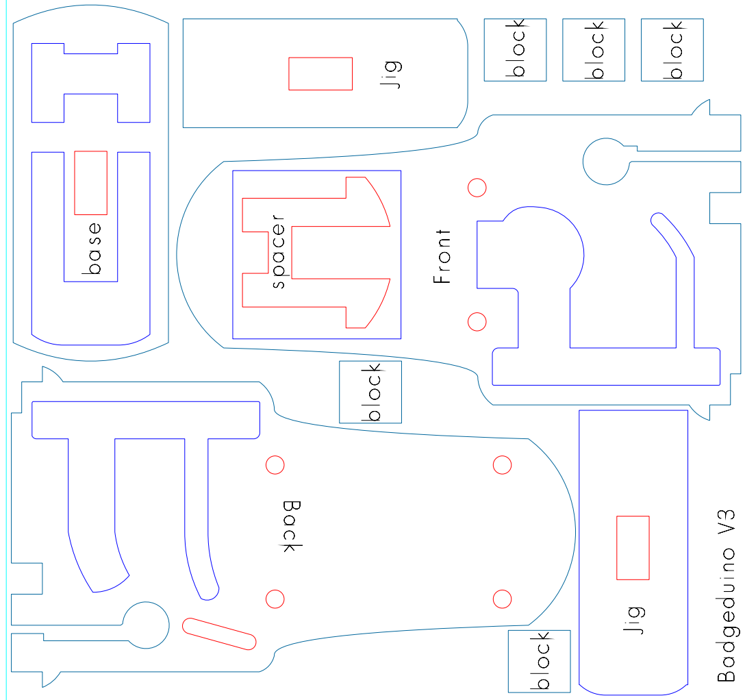
Bodgeduino V3
