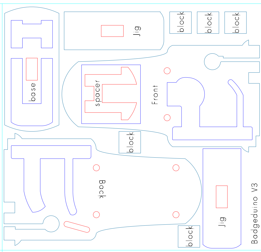
Bodgeduino V3
